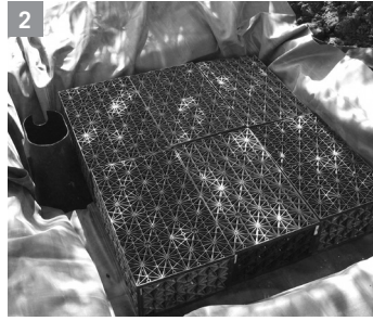
Étape 2 – Installez la voûte Snorkel MC , le module Centipede MC et les matrices d'eau AquaBlox MC
